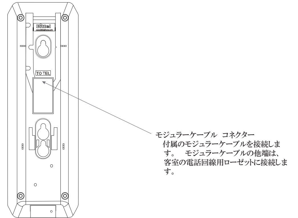
本体 底面図（スタンド取外し時）
