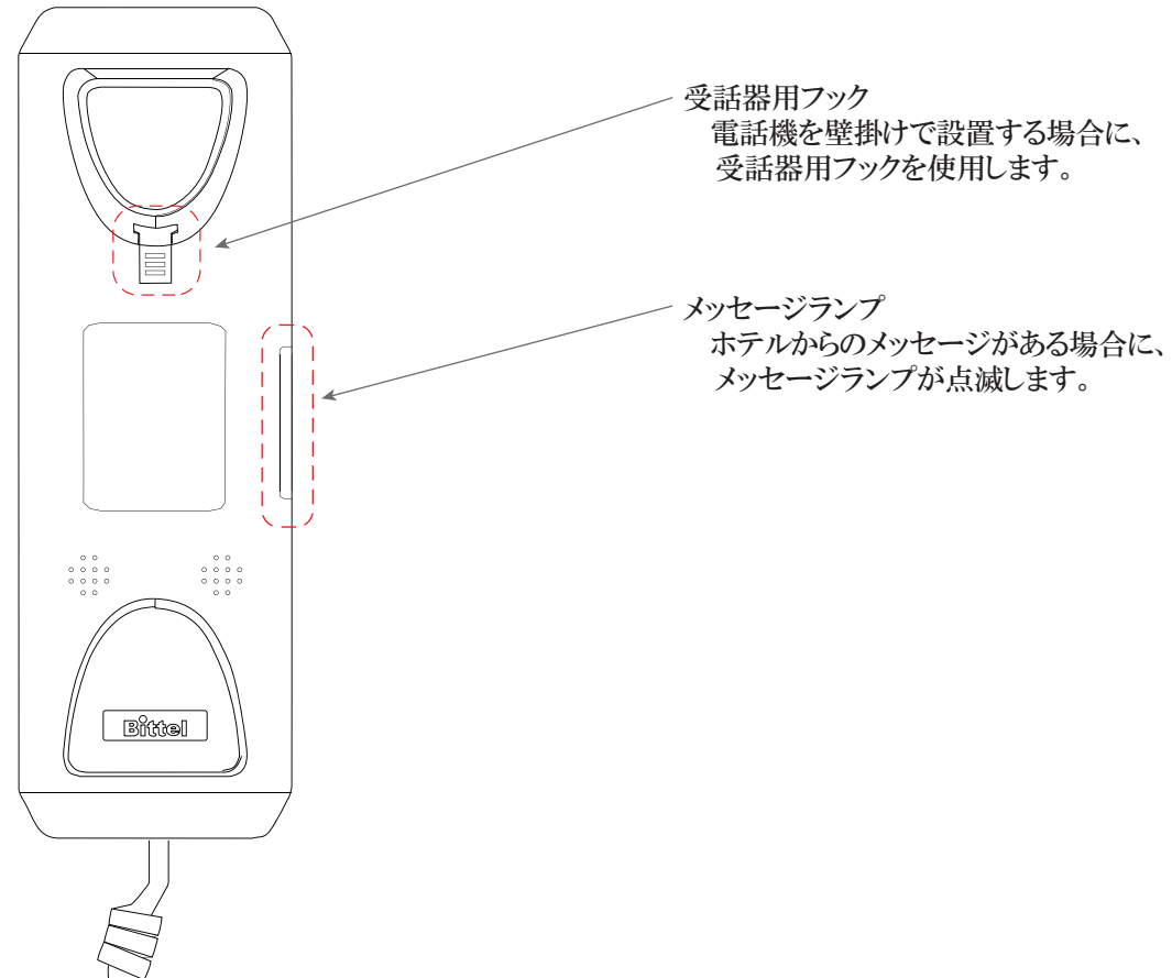
本体 正面図
