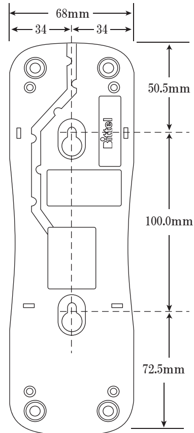
電話機 底面図
